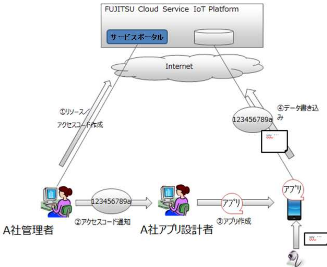
図 3-8. データを書き込みするまでの操作
