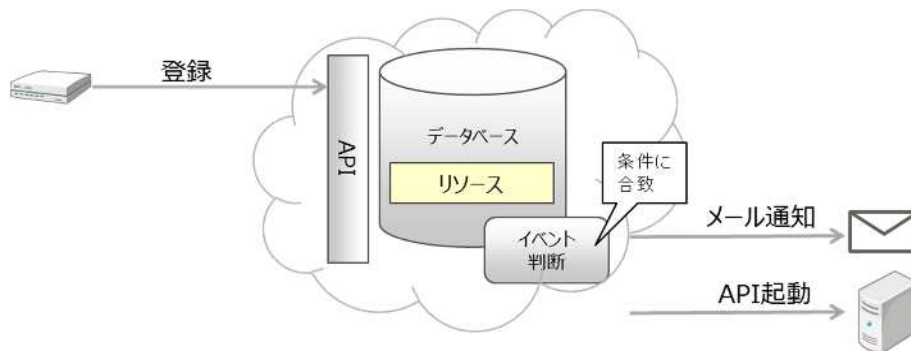
図 3-5. イベント機能
