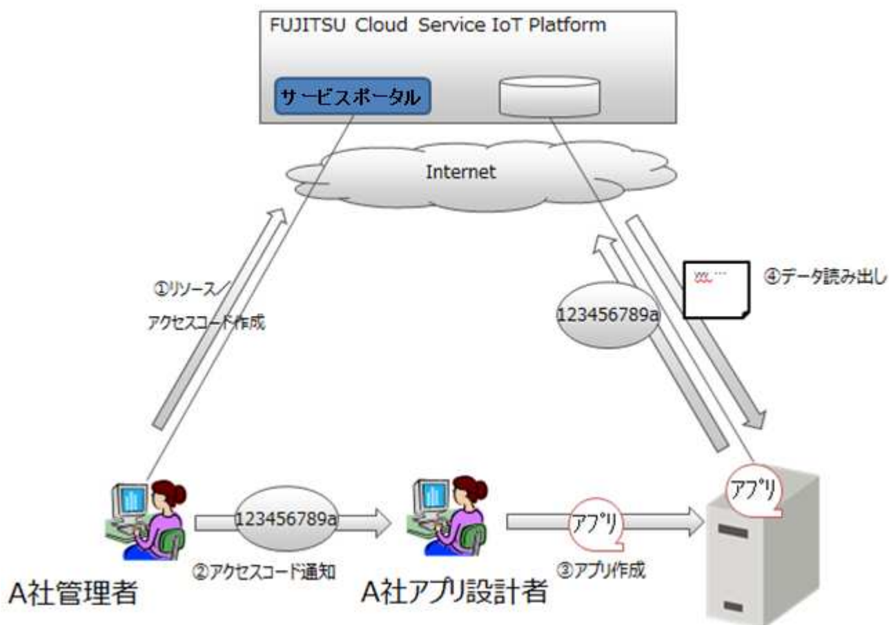
図 3-9. データを参照するまでの操作
